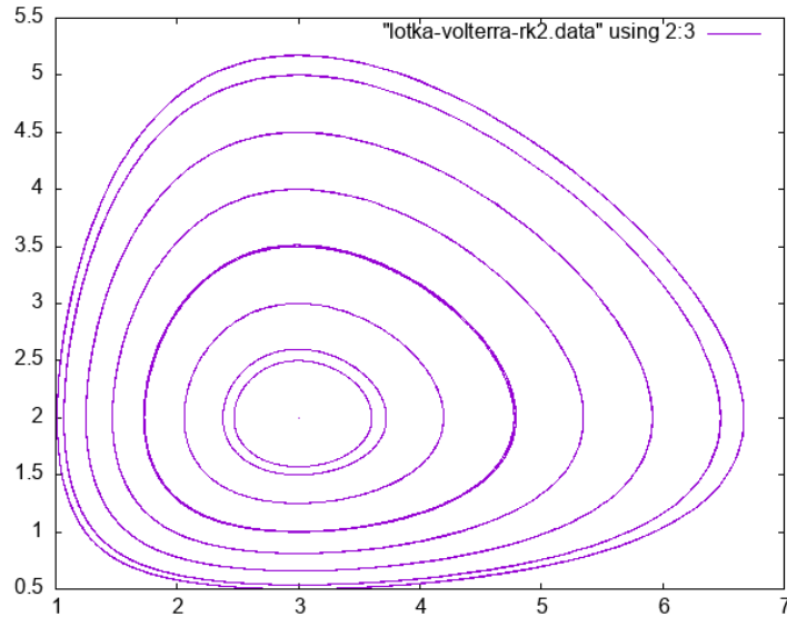
図 20: Lotka-Volterra の方程式の解軌道
