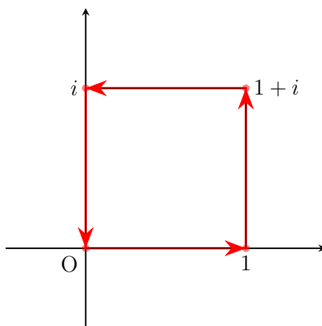
図 15: 正方形の周を正の向きに一周する
