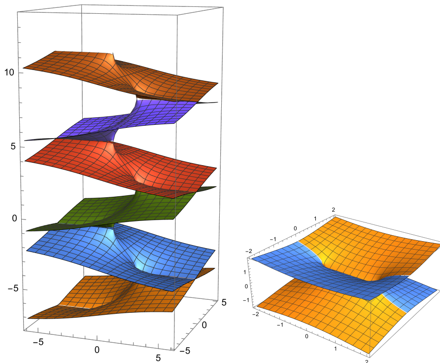
図 12: 実部 (原点のまわりを大きく 3 周分)、虚部はこれで完結
