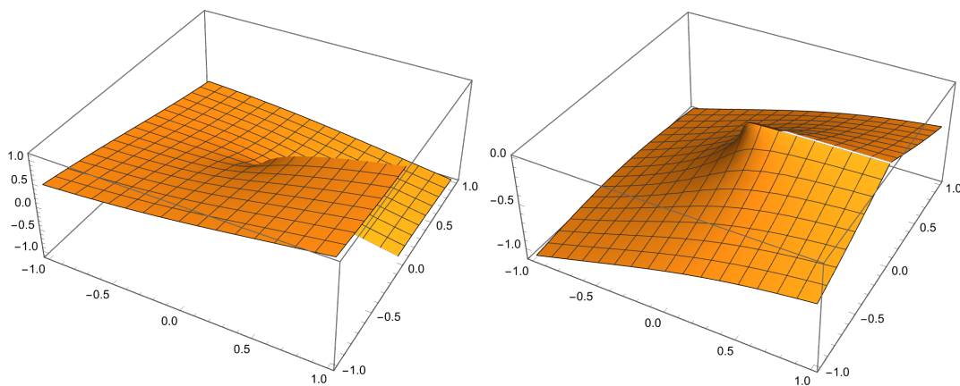
図 7: \operatorname{Re} g のグラフと \operatorname{Im} g のグラフ
