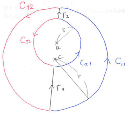
図 20: 切り込みを入れて二つの閉曲線の和として表す
