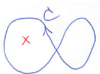
図 34: \int_C f(z) dz \neq 0 かも
