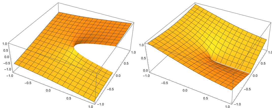
図 6: \text{Re } f のグラフと \text{Im } f のグラフ
