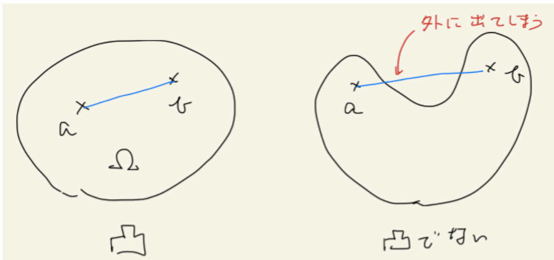
図 18: 凸領域、凸でない領域の典型的イメージ
