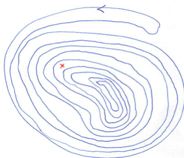
図 38: 曲線 C は赤バツテンの点を囲んでいるか? 即答は難しい。
