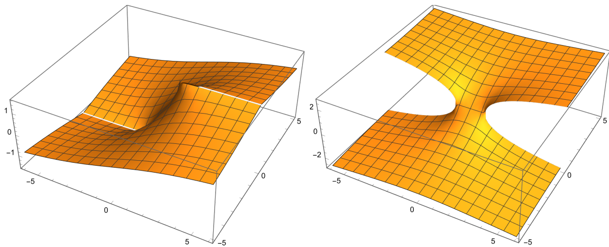
図 9: -i \operatorname{Log} \left( iz + \sqrt{1 - z^2} \right) の実部・虚部のグラフ ( |\operatorname{Re} z| \leq 6, |\operatorname{Im} z| \leq 5 )
