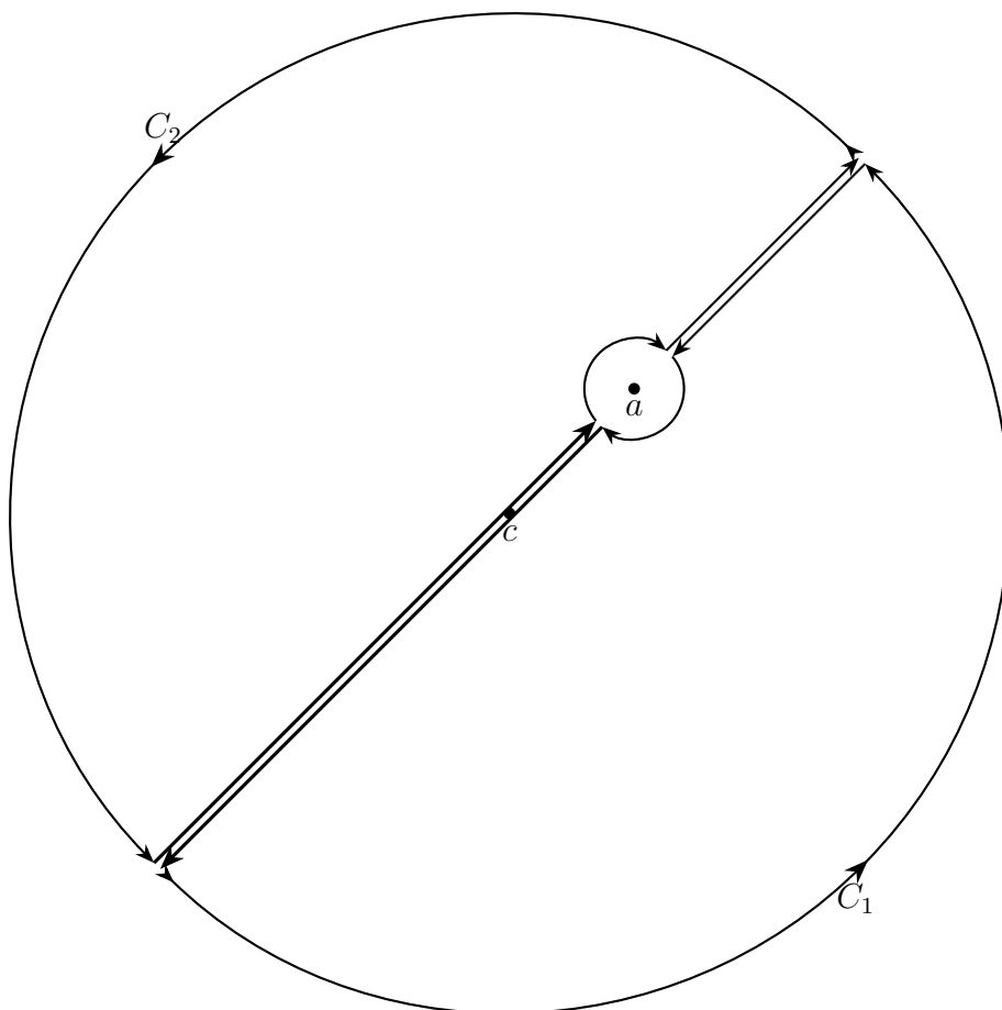
図 27: 証明 3: 2本の橋を渡して、2つの閉曲線を作る
