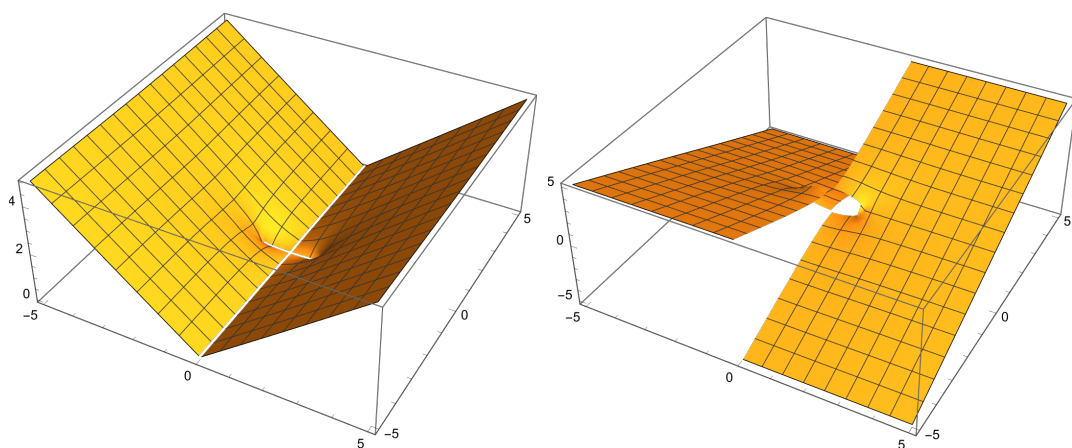
図 13: \text{p.v.}\sqrt{z^2-1} の実部・虚部のグラフ (左半平面で \varphi(z) と異なる)
