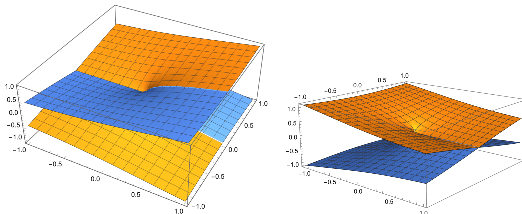
図8: \operatorname{Re} f と \operatorname{Re} g のグラフを重ねる; \operatorname{Im} f と \operatorname{Im} g のグラフを重ねる
