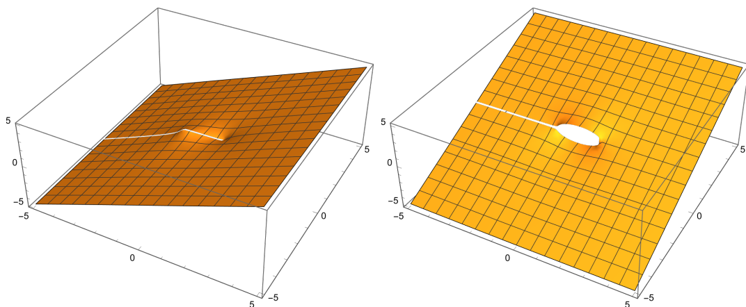
図 14: \varphi(z) = \text{p.v.}\sqrt{z+1} \text{p.v.}\sqrt{z-1} の実部・虚部のグラフ ( [-1, 1] を除けばグラフは滑らか)
