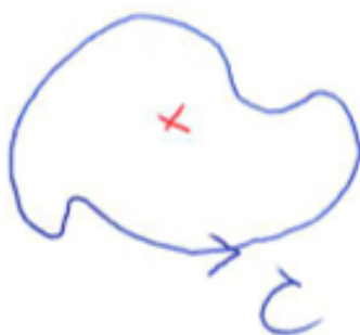
図 33: \int_C f(z) dz \neq 0 かも
