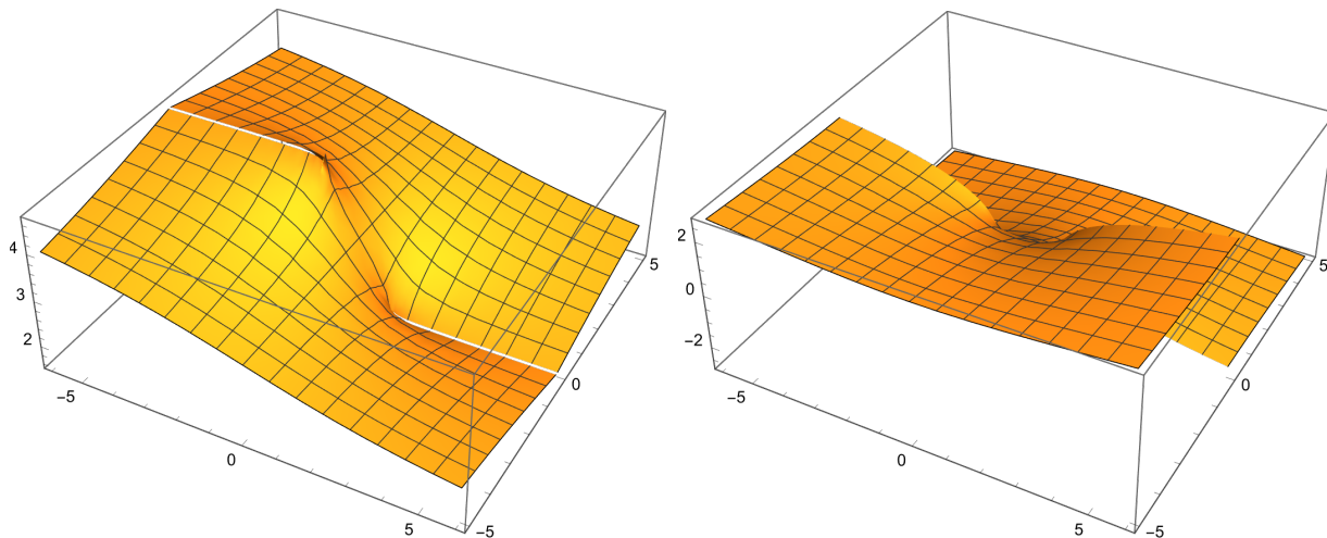
図 11: -i \log_{[0, 2\pi)} \left( iz + \sqrt{1 - z^2} \right) の実部・虚部のグラフ ( |\operatorname{Re} z| \leq 6, |\operatorname{Im} z| \leq 5 )
