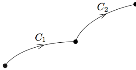
図 16: C_1 の終点 = C_2 の始点ならば C_1 + C_2 が作れる
