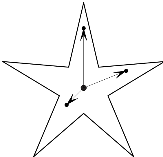
図 19: 星の形は星型領域: ある1点からすべての点が見えるから
