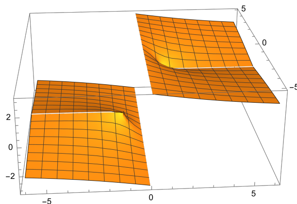
図 10: -i \operatorname{Log} \left( iz - \sqrt{1 - z^2} \right) の実部のグラフ ( |\operatorname{Re} z| \leq 6, |\operatorname{Im} z| \leq 5 )
