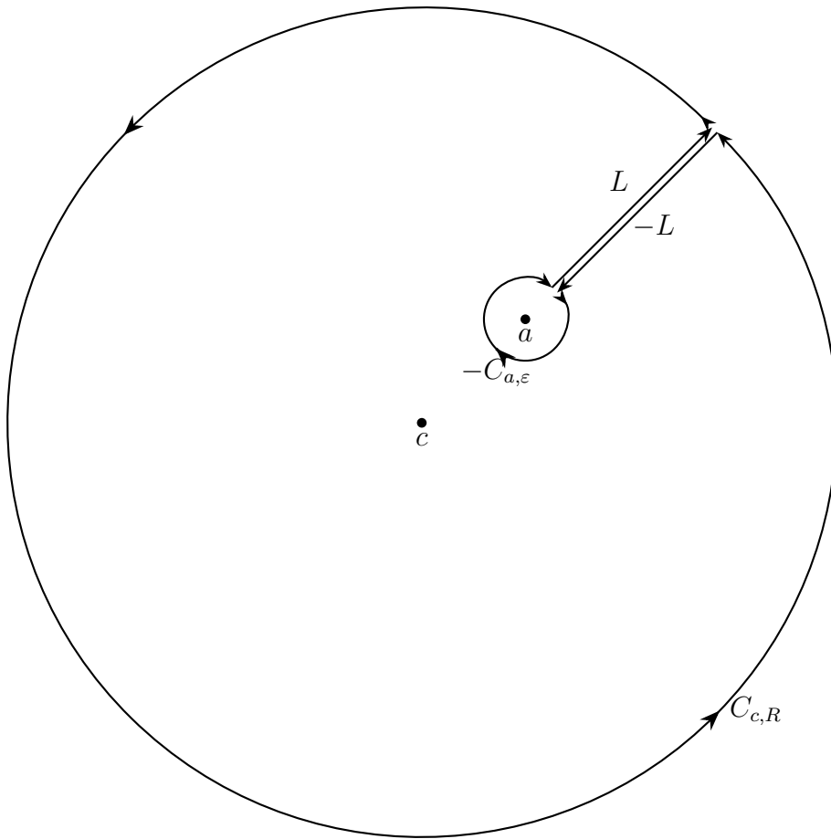
図 25: 証明 1: 1 本の橋 L_\epsilon を渡して a の周りを回って戻る
