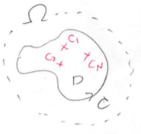
図 31: 特異点 c_j を迂回する積分路 \Gamma を作る
