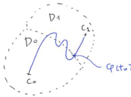
図 30: c_0 から c_1 に至る道、最後に D_0 を出るところ \varphi(t_0)
