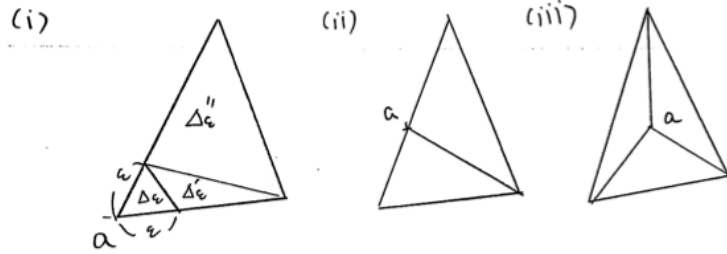
図 17: a が三角形 \Delta のどこにあるかで場合分け (頂点, 辺上, 内部)
