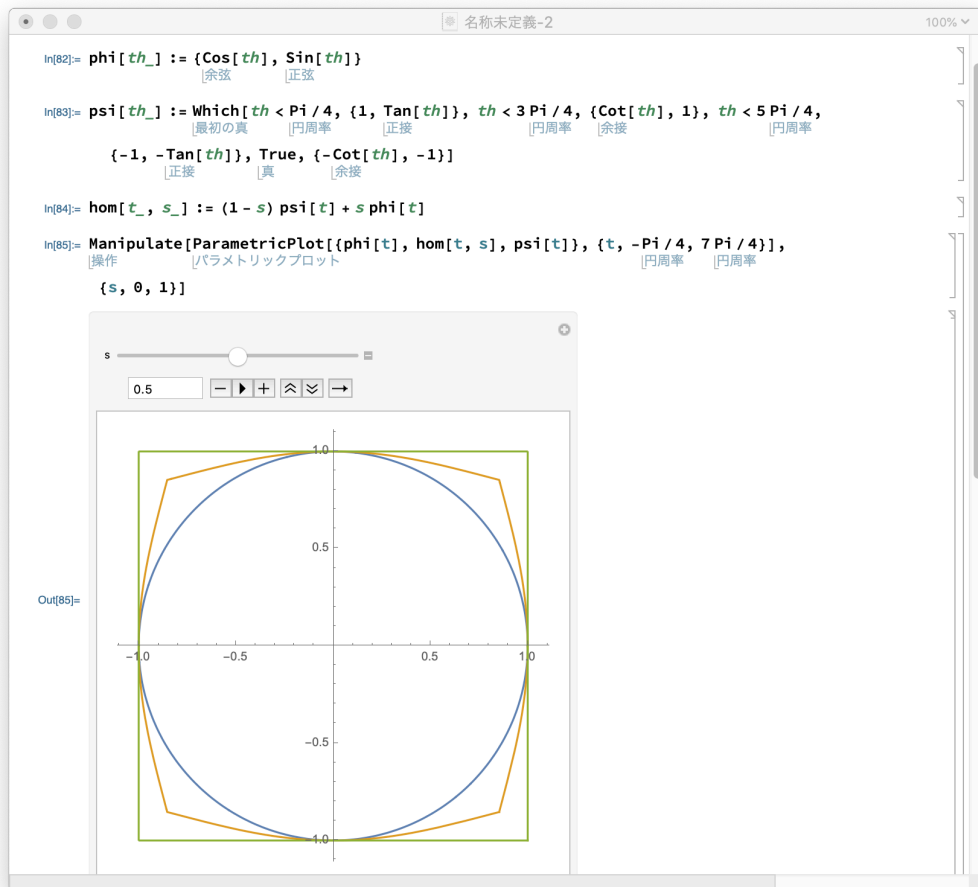
図 29: 正方形の周 \Gamma を円周 C に連続的に変形する
